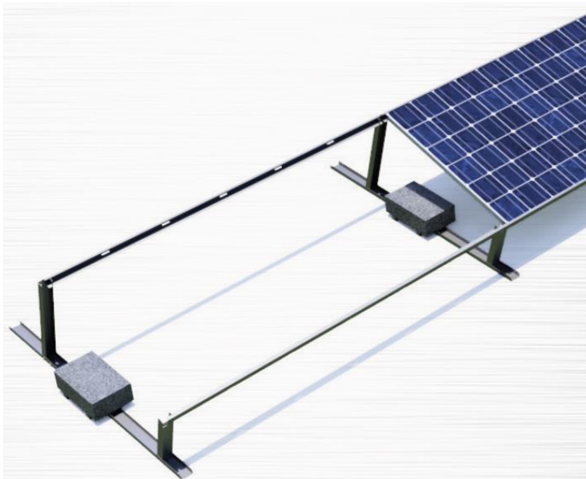
Rys. 1 Widok systemowego mocowania do dachów płaskich przystosowanego do paneli bifacjalnych .
